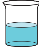
1 mol NaCl
