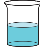
1 mol Sakkaroz
