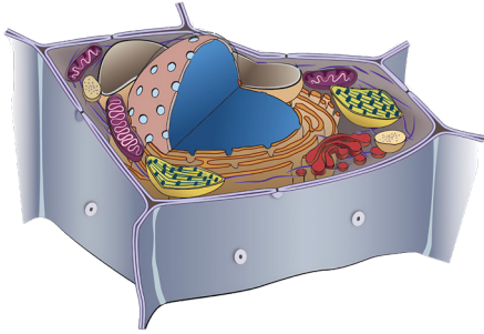
Bitki hücresi
