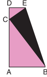
Şekil 2
